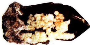
Formation naturelle
