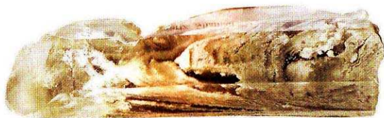
Formation naturelle
