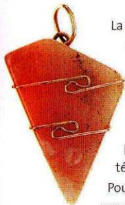
Ussingite
