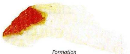
Formation naturelle
