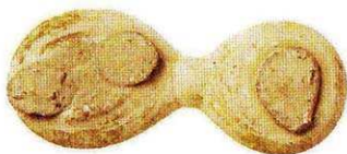
Formation naturelle
