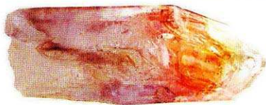
Pointe naturelle
