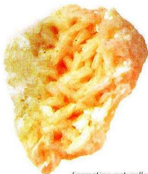
Formation naturelle
