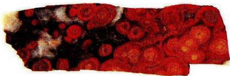
Tranche naturelle
