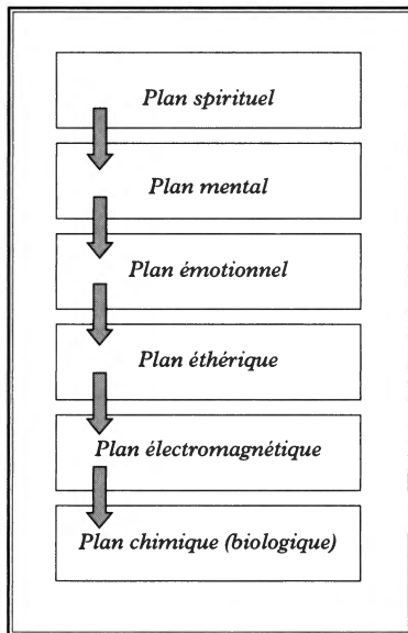
Figure 2.9 Influence des plans supérieurs de réalité.
