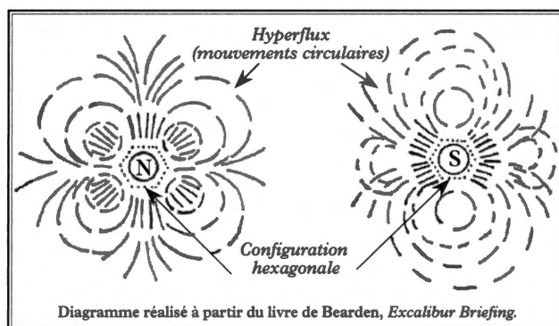
Figure 6.15 Configurations des mouvements circulaires de l'hyperflux magnétique.
