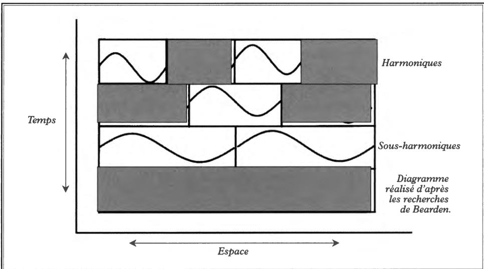
Figure 4.2 Grille de l'espace-temps.
