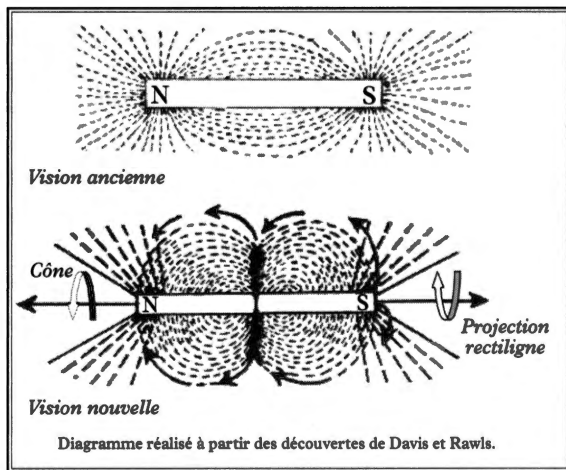
Figure 2.2 Visions ancienne et nouvelle du magnétisme.
