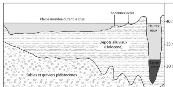
Fig. 3.1 Coupe de la vallée du Nil en Haute-Égypte
