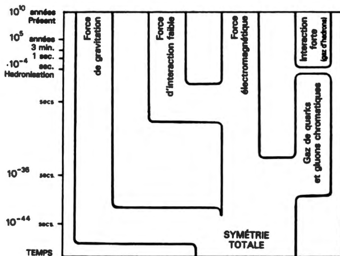
Figure 17.1 Arbre évolutif des champs de la nature sous-tendant les quatre types de force connus. Selon les théories du champ modernes, au début des temps, les champs de la nature, qui nous apparaissent aujourd'hui distincts, étaient unis ; les champs connus de la physique sont apparus par ruptures de symétrie successives (d'après Pagels, 1985).
