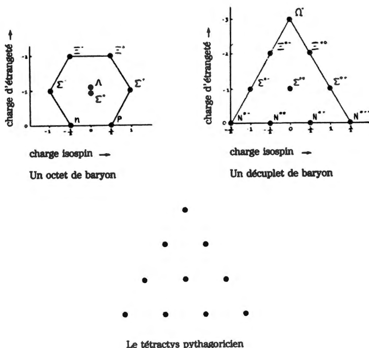
Figure 2.2 Deux familles de baryon (d'après Pagels, 1983). Les baryons sont des particules élémentaires de spin demi-entier participant à des interactions fortes. Chacun contient trois quarks, qui se présentent selon trois «couleurs»: haut , bas et étrange . Les différents types de baryon contiennent des combinaisons caractéristiques de quarks; par exemple le proton a deux haut et un bas , et le neutron a un haut et deux bas . L'octet de baryon est souvent appelé «la voie octuple». Le décuplet de baryon est organisé à la manière du tétractys, l'antique symbole qui réside au cœur de la sagesse des nombres de Pythagore.
