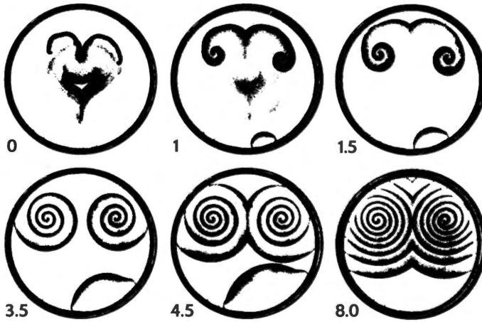
Figure 5.7 La formation d'ondes chimiques en spirale quand le réactif Belousov-Zhabotinski est livré à lui-même dans une coupelle creuse. Les ondes apparaissent spontanément au fil de la réaction chimique, ou peuvent être stimulées en touchant la surface avec un filament chaud, comme dans les illustrations ci-dessus. Les chiffres indiquent le nombre de secondes s'étant écoulées après la photographie initiale (adapté de From Being to Becoming , avec l'autorisation d'Ilya Prigogine, copyright 1980, W. H. Freeman and Co.).
