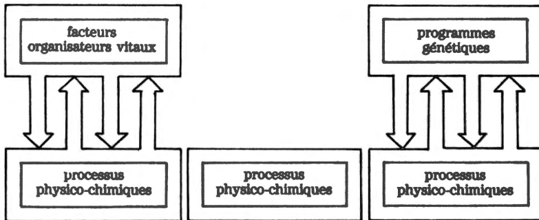
Figure 5.5 À gauche, diagramme illustrant la théorie vitaliste : les processus physico-chimiques inhérents aux organismes interagissent avec – et sont organisés par – des facteurs organisateurs vitaux, tels que l'entéléchie. La théorie mécaniste nie l'existence de tels facteurs vitaux, et prétend que la vie n'est compréhensible qu'en termes de processus physico-chimiques (centre). Dans la conception moderne (droite), ces processus sont organisés par des programmes génétiques ou par une information génétique, jouant sensiblement le même rôle que les facteurs organisateurs du vitalisme.
